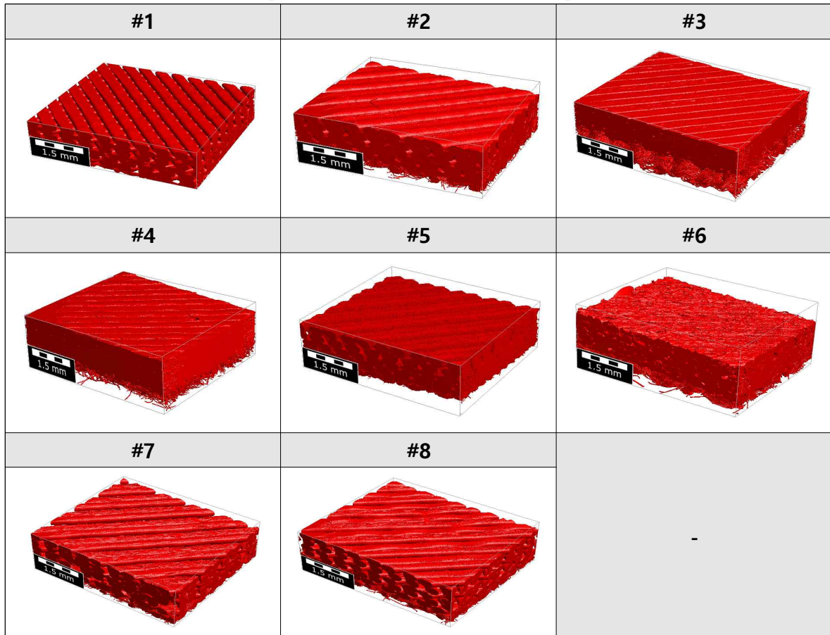
[부직포의 XRM 기반 모델 형상]
