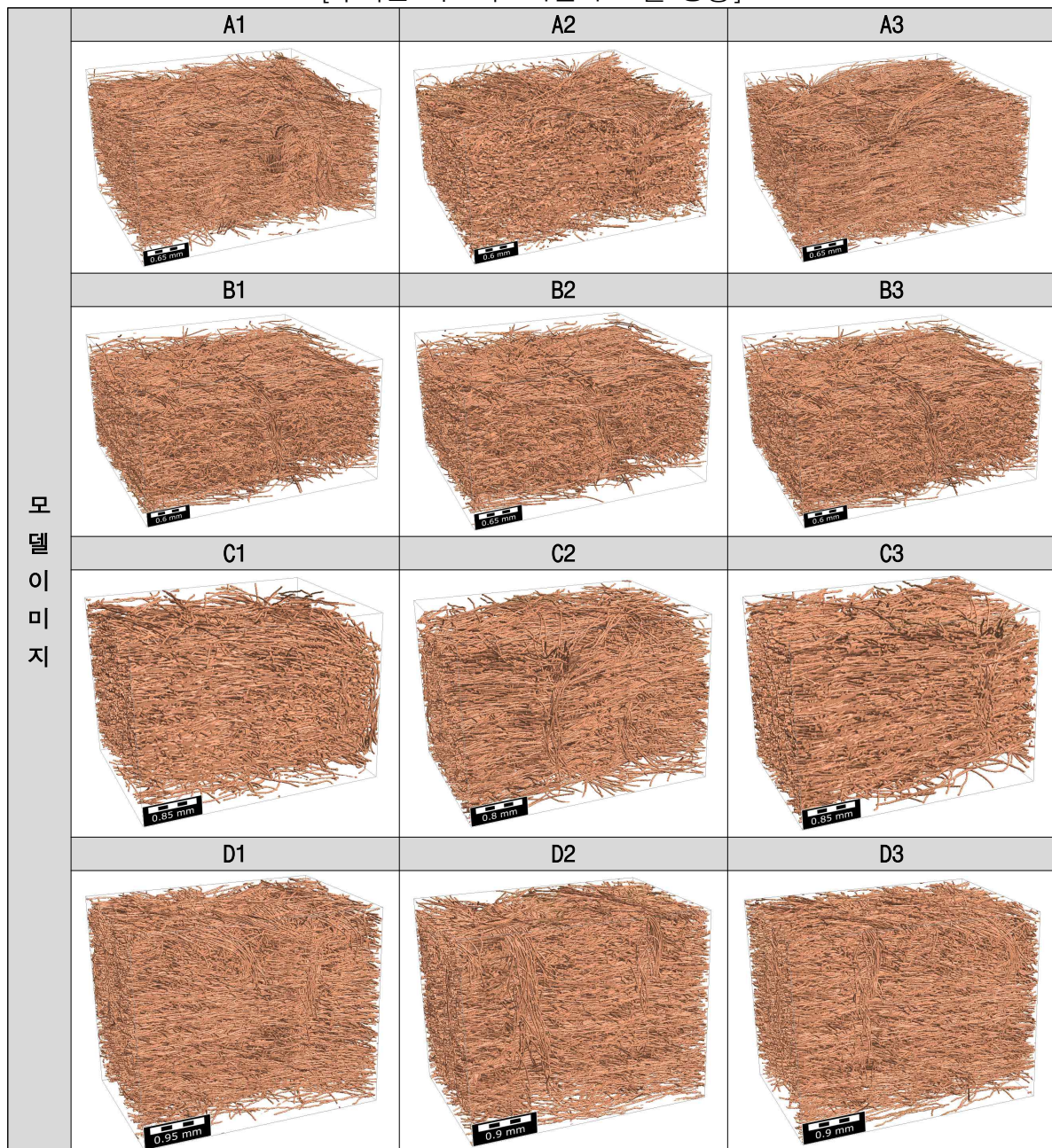
[구축된 지오텍스타일의 모델 형상]
