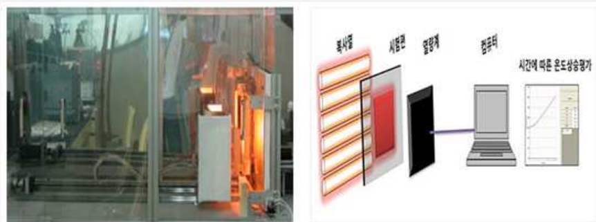
< 복사열 통과량 시험 장비 >
